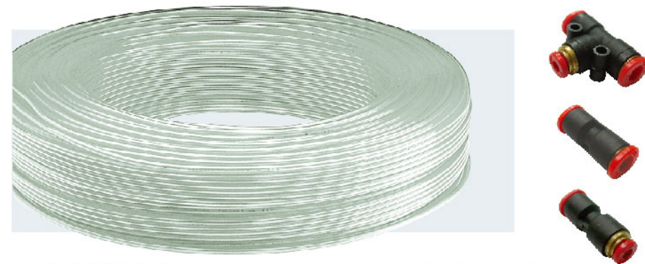
FT-4: 4公釐的液體導管 FT-6: 6公釐的液體導管 FLF-4: 連接 4公釐液體導管的濾嘴 FLF-6: 連接 6公釐液體導管的濾嘴
